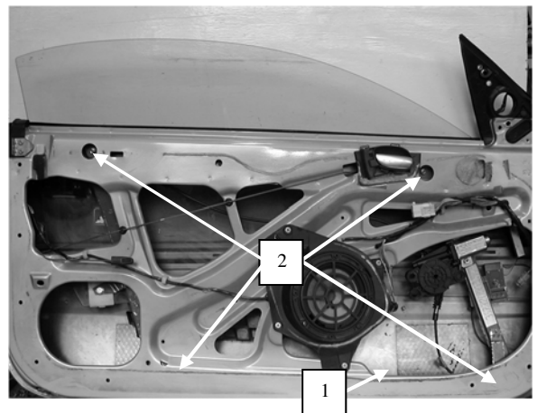
Porta lato sinistro, Portière avant gauche, Left front door, Puerta lado izquierdo, Vorne links Tür, Porta frente esquerda, Sol on kapi, πόρτα εμπρόςθια αριστερή
