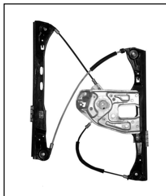
Alzacristallo originale – oem window regulator – lève-vitre original – Fensterheber von oem – elevalunas original – levandator de vidro original – orijinal cam acacagi - Γρύλος νησίσιος
