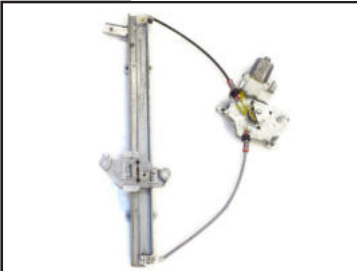
Alzacristallo originale - oem window regulator - lève-vitre original - Fensterheber von oem - elevallunas original - levantator de vidro original - orijinal cam acacagi - Γρύλος γνήσιος
