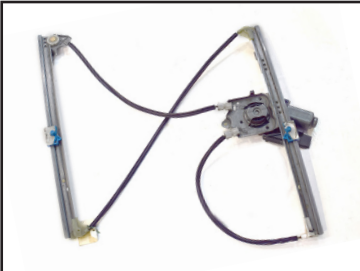
Alzacristallo originale - oem window regulator - lève-vitre original - Fensterheber von oem - elevalunas original - levantator de vidro original - orijinal cam acacagi - Γρύλος γνήσιος
