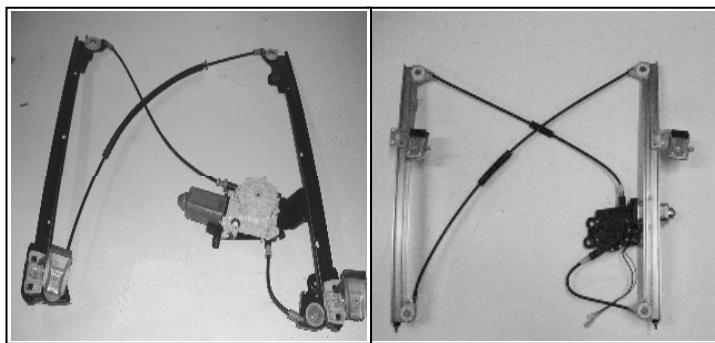
Alzacristallo originale – oem window regulator – lève-vitre original – Fensterheber von oem – elevaunas original – levantador de vidro original orijinal cam acacagi - Γρύλος γνήσιος
